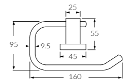
Toilet roll holder 2261350
